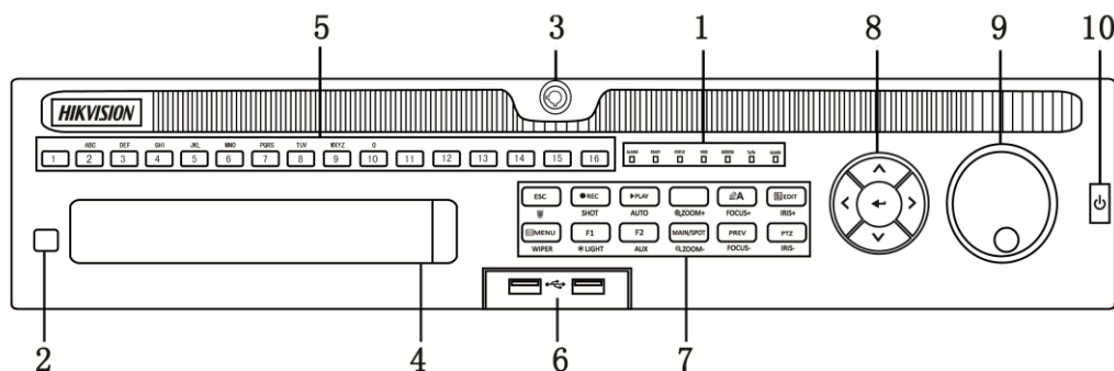
Figure 1. 7 Panneau avant du DS-9000HQHI-SH
