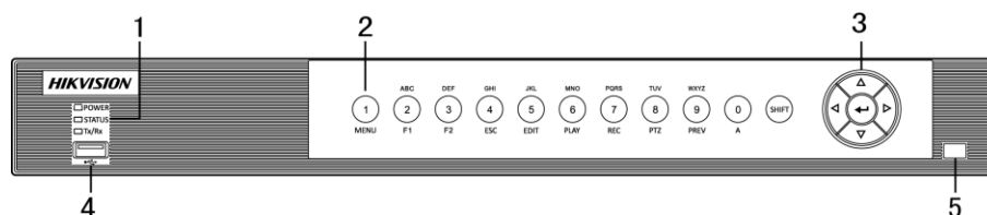
Figure 1. 4 Panneau avant du DS-7200HQHI-SH
