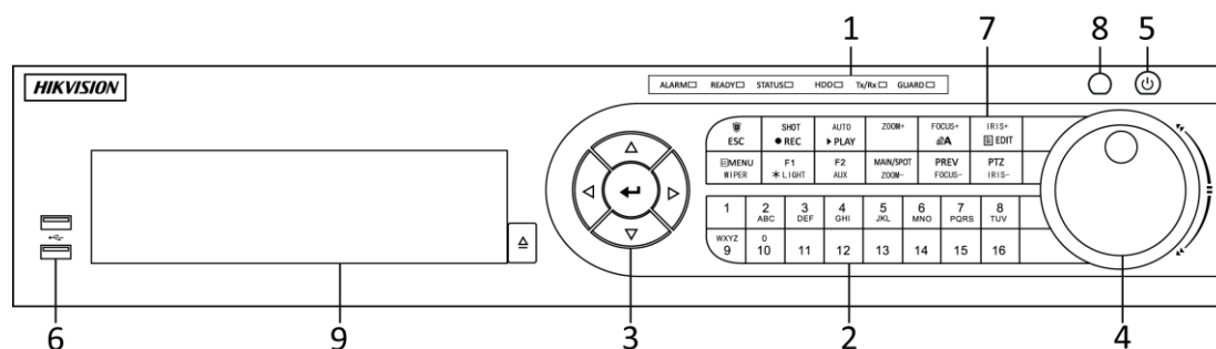
Figure 1. 6 Panneau avant du DS-8100-SH
