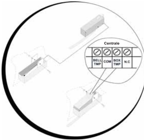
Figure 10: Raccordement du contact d'autoprotection du boîtier
