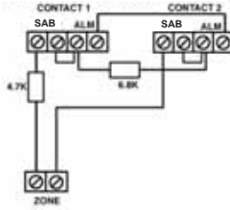
SCHEMA DE CABLAGE DE ZONE DEOL POUR DOUBLE PORTE
