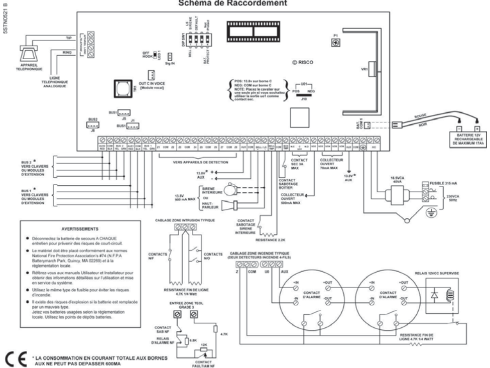
Figure 4 : Schéma de Raccordement de la Carte Mère
