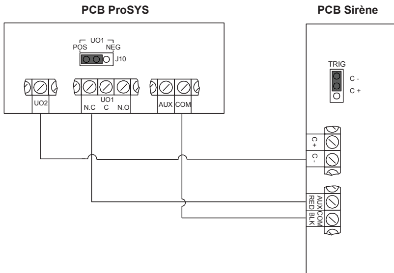
Figure 9: Câblage de la sirène : Configuration C-
