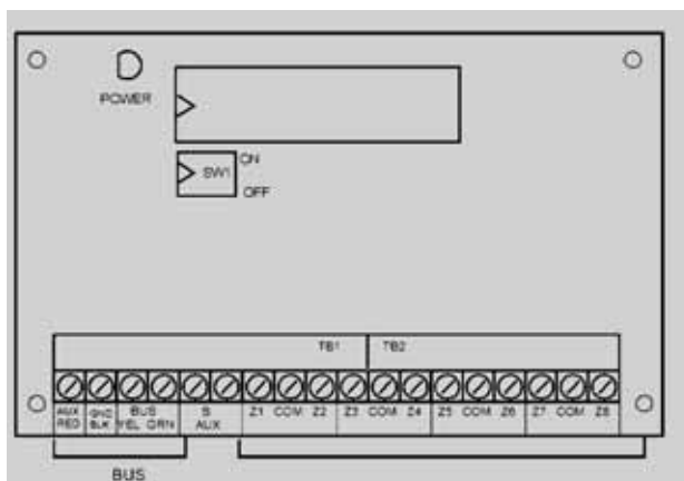
Figure 17: Module d'Extension de Zones ZE8 (Exemple d'un câblage zone typique)
