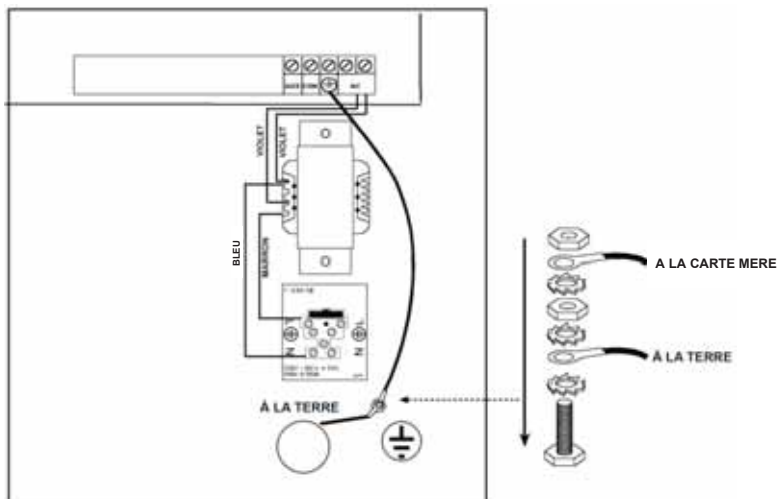
Figure 12 : Raccordement à la Terre du Boîtier Métallique
