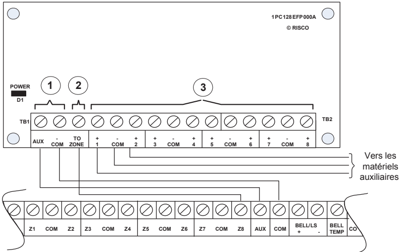
Figure 7: Bornier de la Carte Mère
