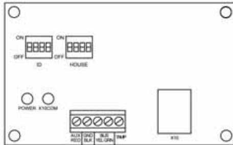
Figure 21 : Module d'Extension X-10
