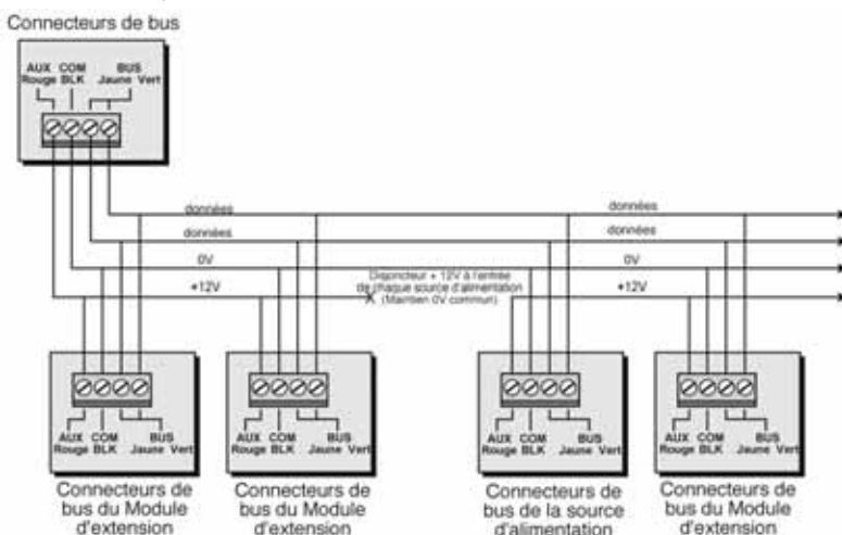
Figure 5 : Extension de BUS à 4 fils
