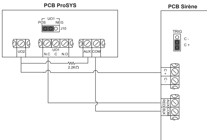
Figure 8 : Câblage de la sirène : Configuration C+
