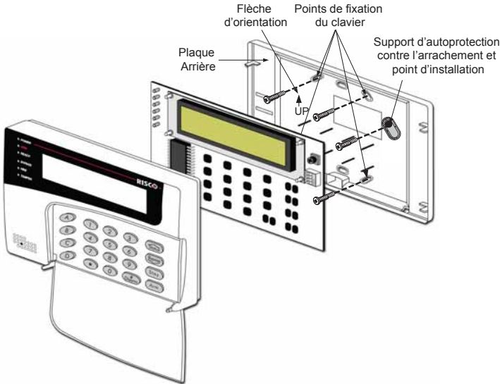
Figure 16: Vue de face de l'Installation du Clavier
