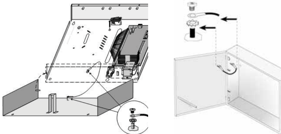
Figure 12 : Raccordement à la Terre du Boîtier Métallique
