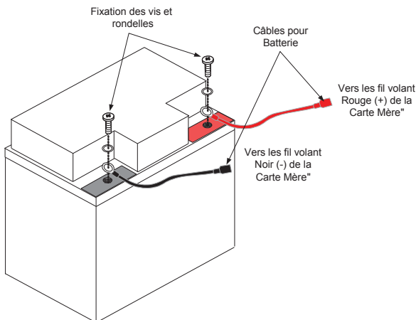
Figure 14 : Connexion d'une batterie 12V/17Ah
