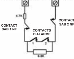
CONFIGURATION ZONE DEOL POUR DOUBLE PORTE
